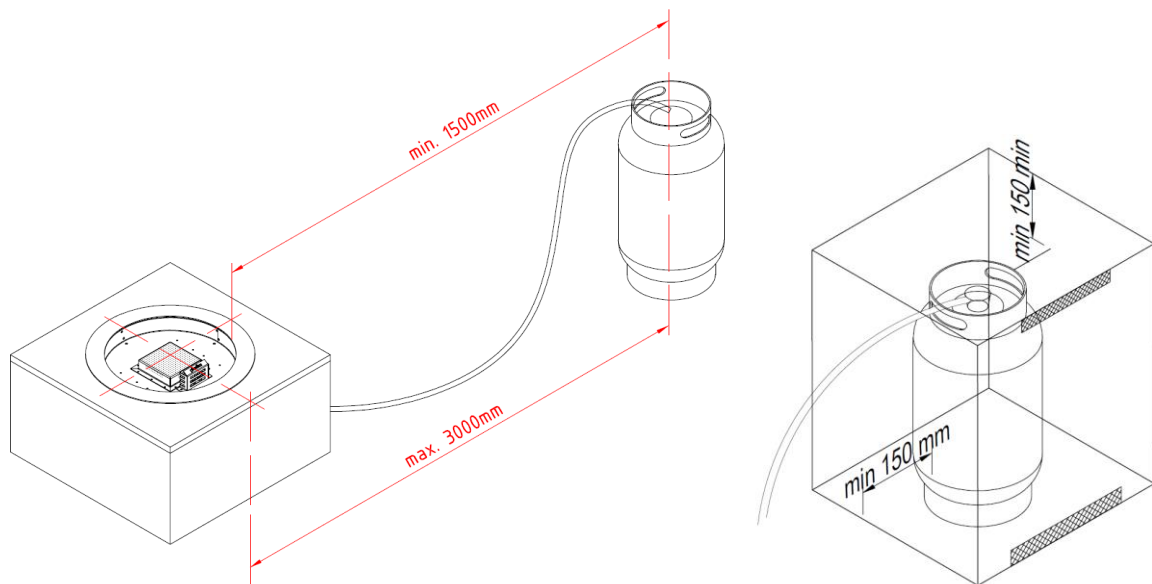
Abbildung 3 – Abstand zwischen der Feuerstelle und Gasflasche sowie Gasflaschenverkleidung
