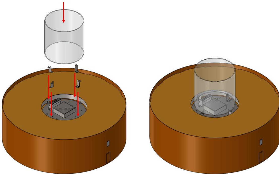
Abbildung 2 – Montage des Glaszylinders
