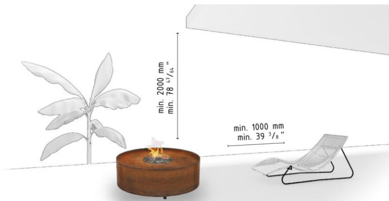
Abbildung 1: Mindestabstand zu brennbaren Materialien
